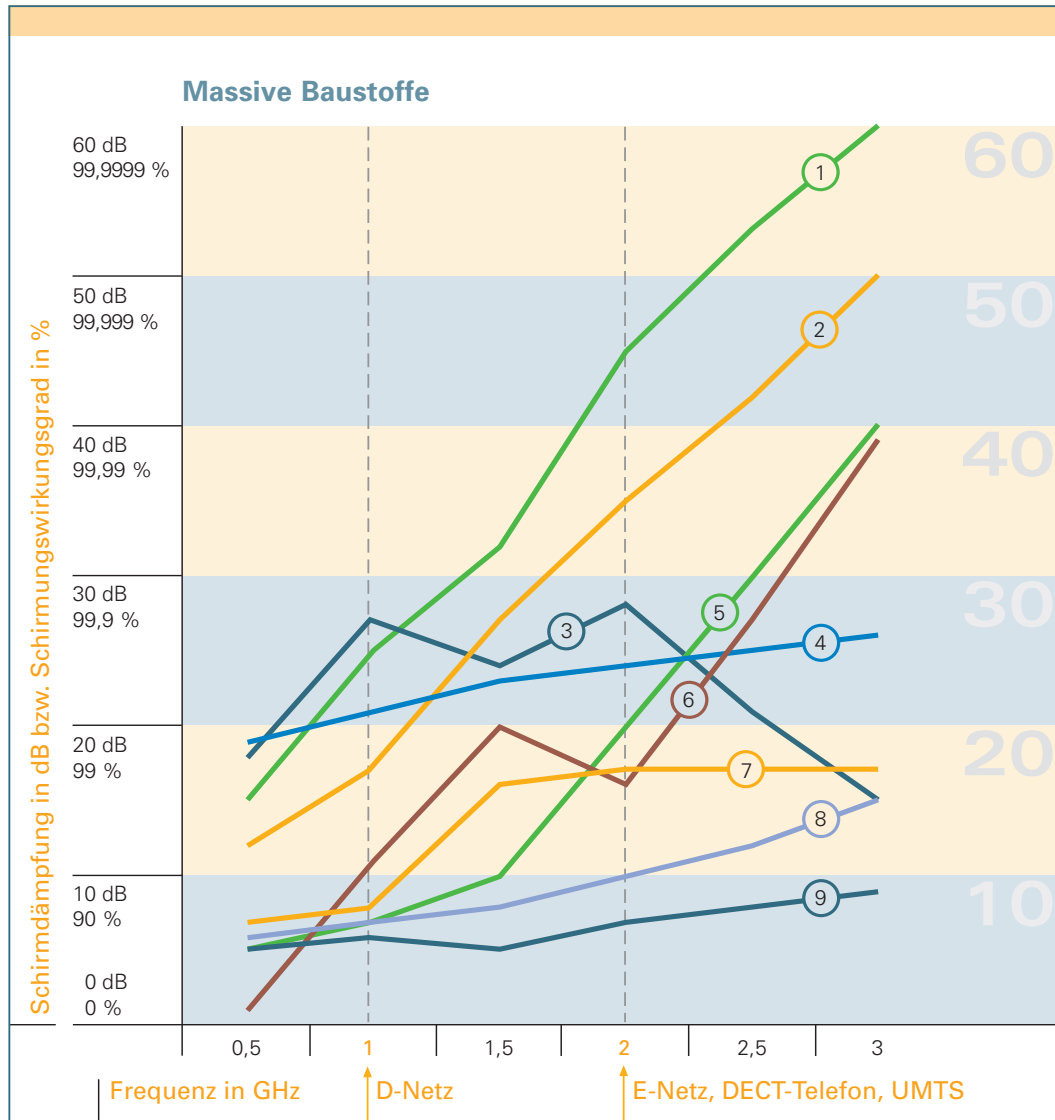
Abb. 10: Messergebnisse für die Schirmung massiver Baustoffe
